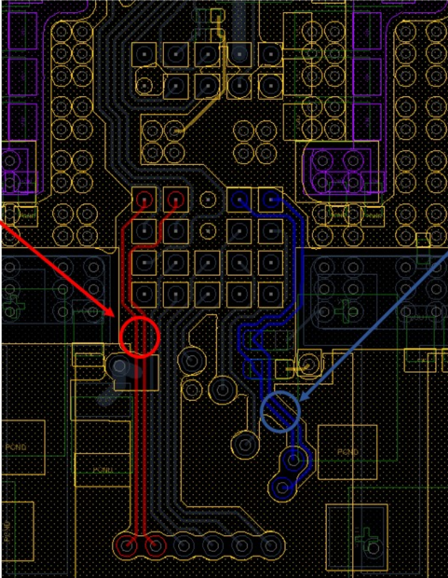
Figure 33 : VSense Traces
